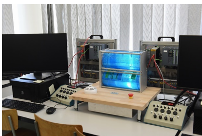
Zdjęcie nr 2 laboratorium (stan na dzień 18.04.2019r.)
